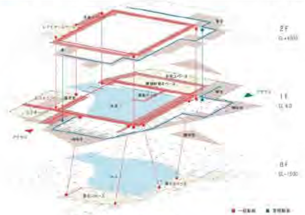
図6) 動線計画
