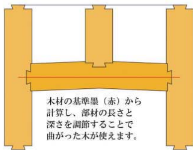
芯基準の図(大工)
