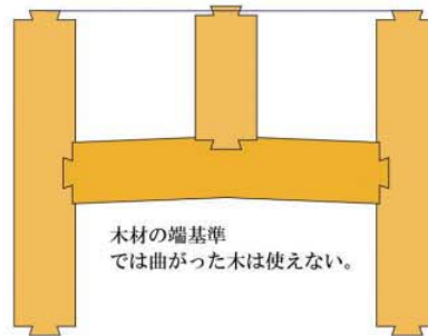
端基準の図(工場)
